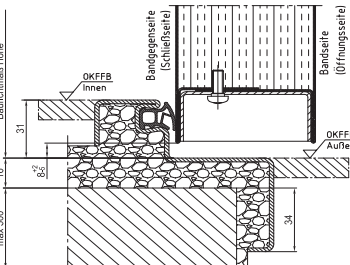
B2 Schwelle für kleine Türen bis BRM-Höhe 1749 mm und Türen ab BRM-Höhe 1750 mm 4-seitig umlaufender Rahmen (Zarge 4-seitig umlaufend) 3)
