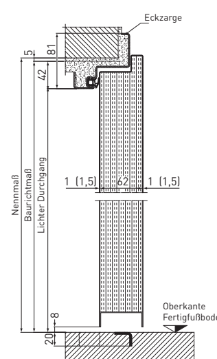
Vertikalschnitt
