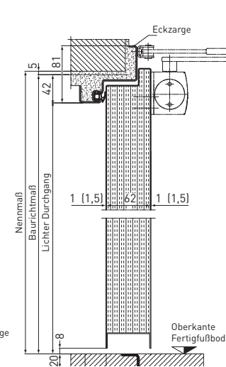
Vertikalschnitt
