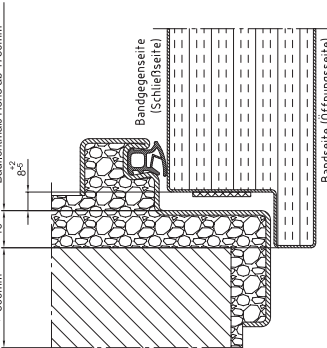
B1 Schwelle für Türen mit 4-seitig umlaufenden Rahmen (Türblatt und Zarge 4-seitig umlaufend)
