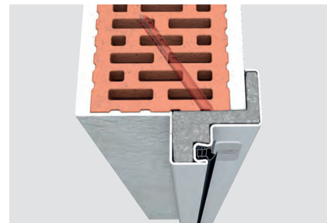
EI 2 30, MZ
