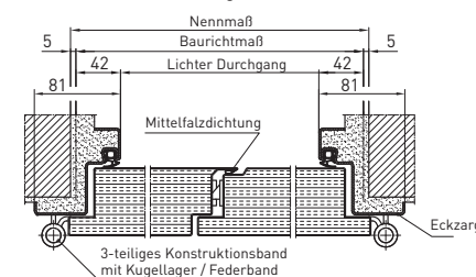
Horizontalschnitt 2-flgl.
