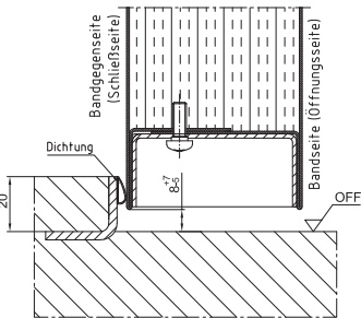
C2 Schwelle mit unterem Anschlag und Dichtung 2)
