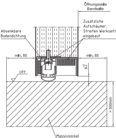
B1 Schwelle für Wandklappen mit 4-seitig umlaufenden Rahmen (Türblatt und Zarge 4-seitig umlaufend)
