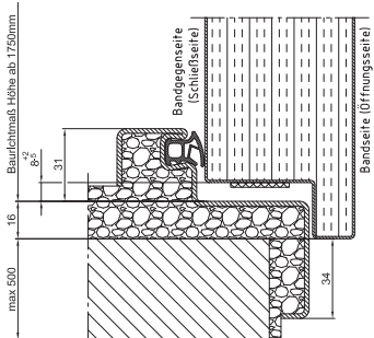
B1 Schwelle für Türen ab BRM-Höhe 1750 mm 4-seitig umlaufender Rahmen (Türblatt und Zarge 4-seitig umlaufend)
