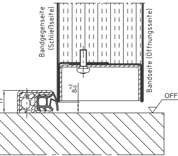
BE-2 Schwelle mit 4-seitig umlaufendem Rahmen
