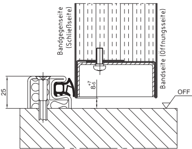
B3 Schwelle mit 4-seitig umlaufendem Rahmen
