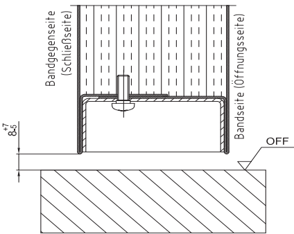
B2 Schwelle für kleine Türen bis BRM-Höhe 1749 mm und Türen ab BRM-Höhe 1750 mm 4-seitig umlaufender Rahmen (Zarge 4-seitig umlaufend) 3)
