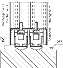
2xRS1 doppelt absenkbare Bodendichtung 2)
