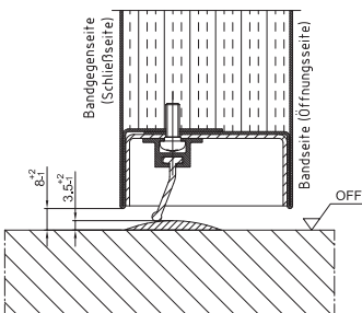
RS2 Dichtungsschwelle/Höckerschwelle 1)2)
