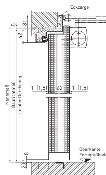
Vertikalschnitt
