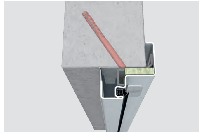
EI 2 30, MZ
