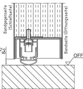
RS1/RS1V absenkbare Bodendichtung
