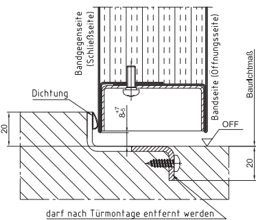
RS2 Dichtungsschwelle/Höckerschwelle 1)2)
