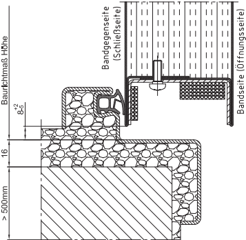
B2 Schwelle mit 4-seitig umlaufenden Rahmen (Zarge 4-seitig umlaufend / Türblatt 3-seitig 2)
