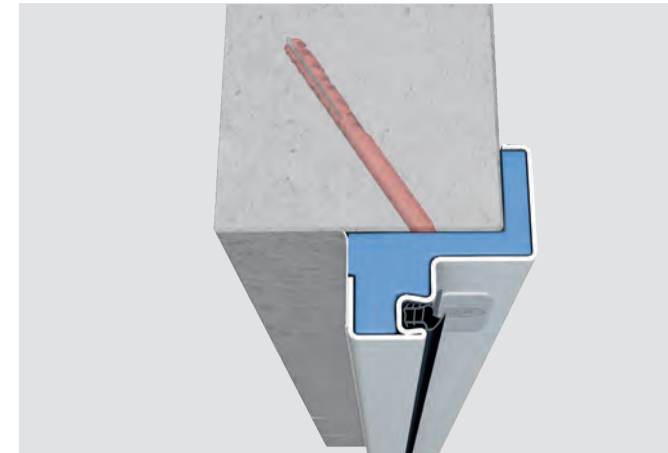
EI 2 30, MZ
