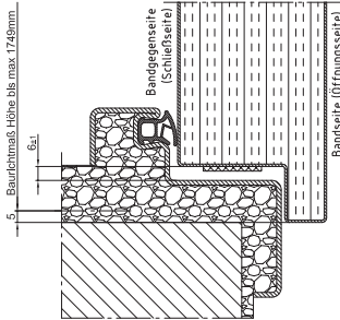
B1 Schwelle nur für Wandklappen bis BRM-Höhe 1749 mm 4-seitig umlaufender Rahmen (Türblatt und Zarge 4-seitig umlaufend)
