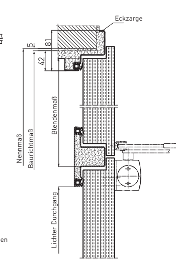
Vertikalschnitt mit Oberblende
