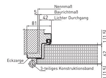
Horizontalschnitt 2-flgl.
